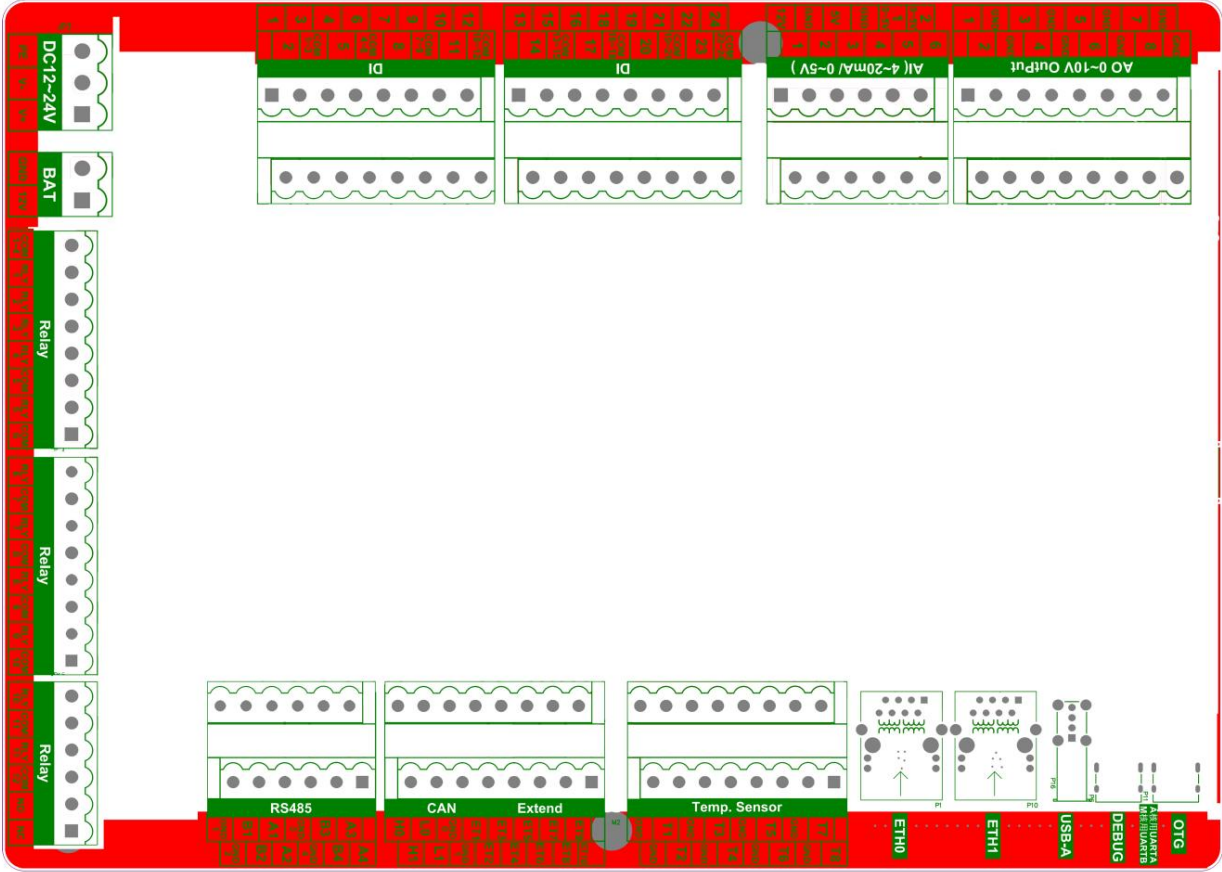
图 1-1 JXYJY-PLC-37 局部布板图
