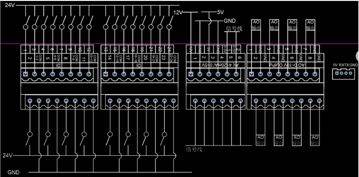
图 2-2 JXYJY-PLC-37 (左 DI、中 AI、右 AO)接线图
