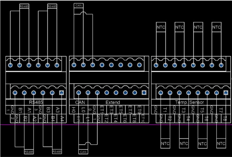
图 2-4 JXYJY-PLC-37 (左 RS485、中 CAN、右 NTC)接线图
