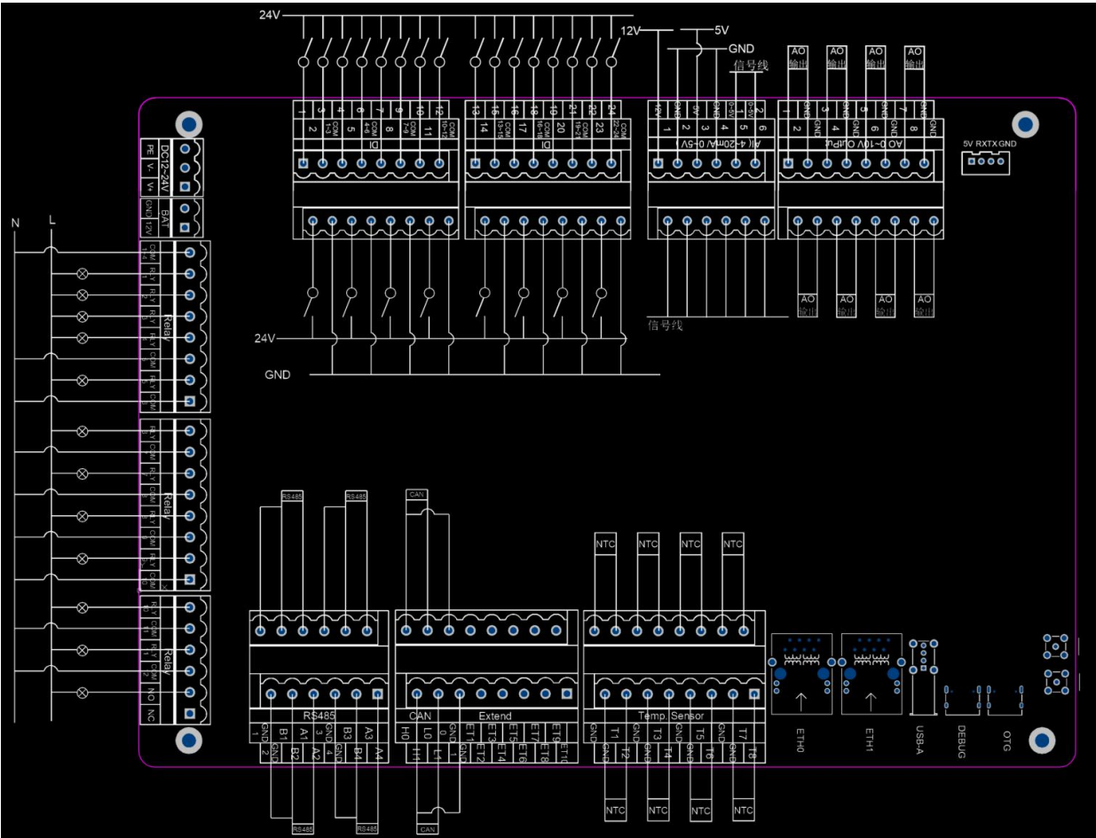
图 2-1 JXYJY-PLC-37 整体接线图
